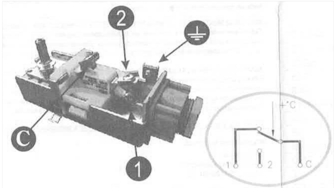
Schéma de raccordement
