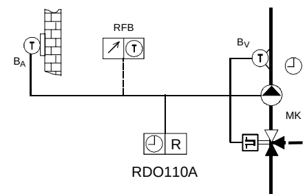
Circuit de chauffage avec vanne mélangeuse 2 points (vanne thermique)
